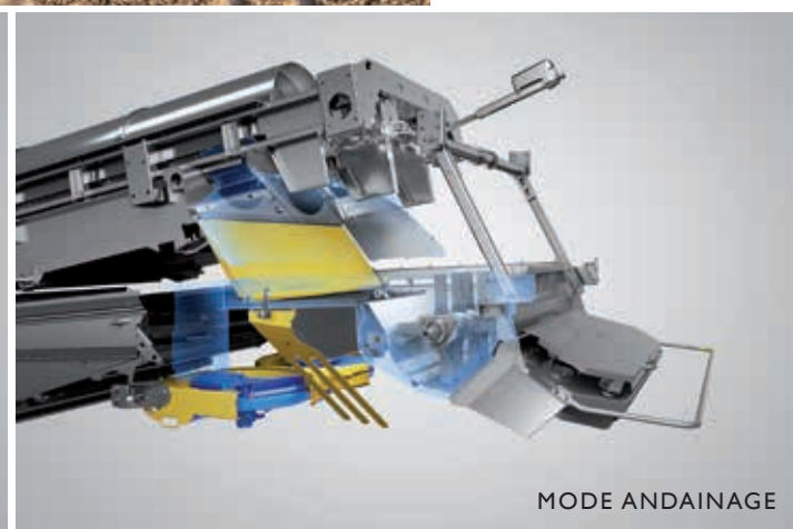
MODE BROYAGE
