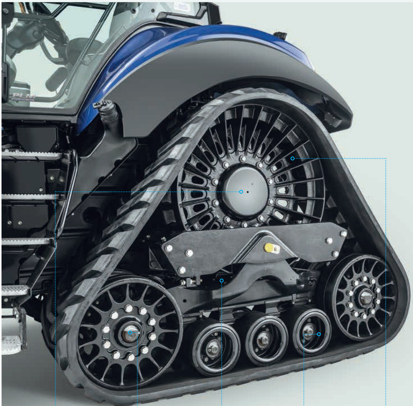
Roue motrice de grand diamètre en fonte ductile
